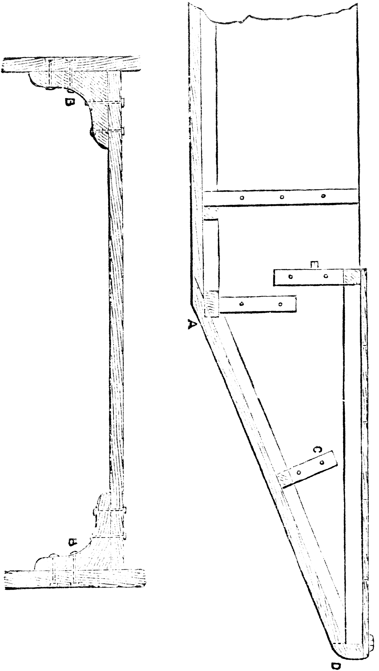
FIG. 16. END AND DECKING OF PUNT.
