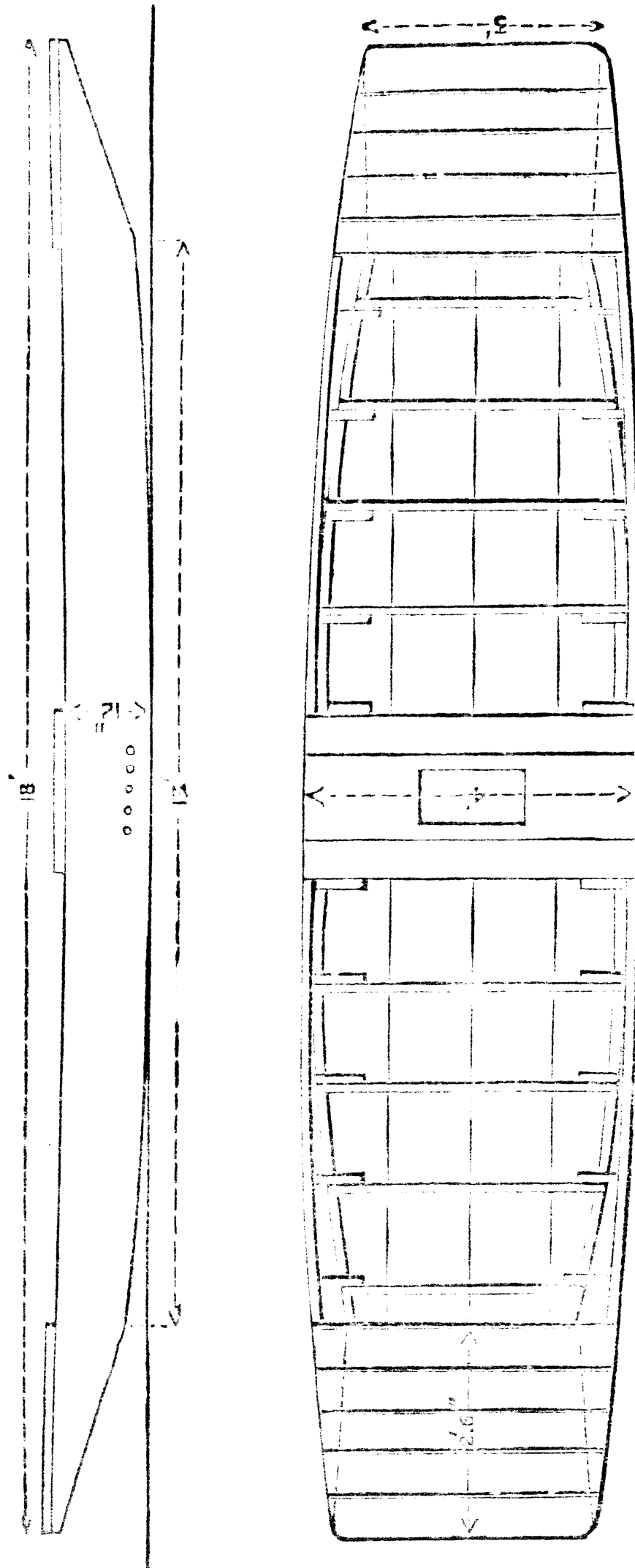
FIG. 12. FISHING PUNT.
